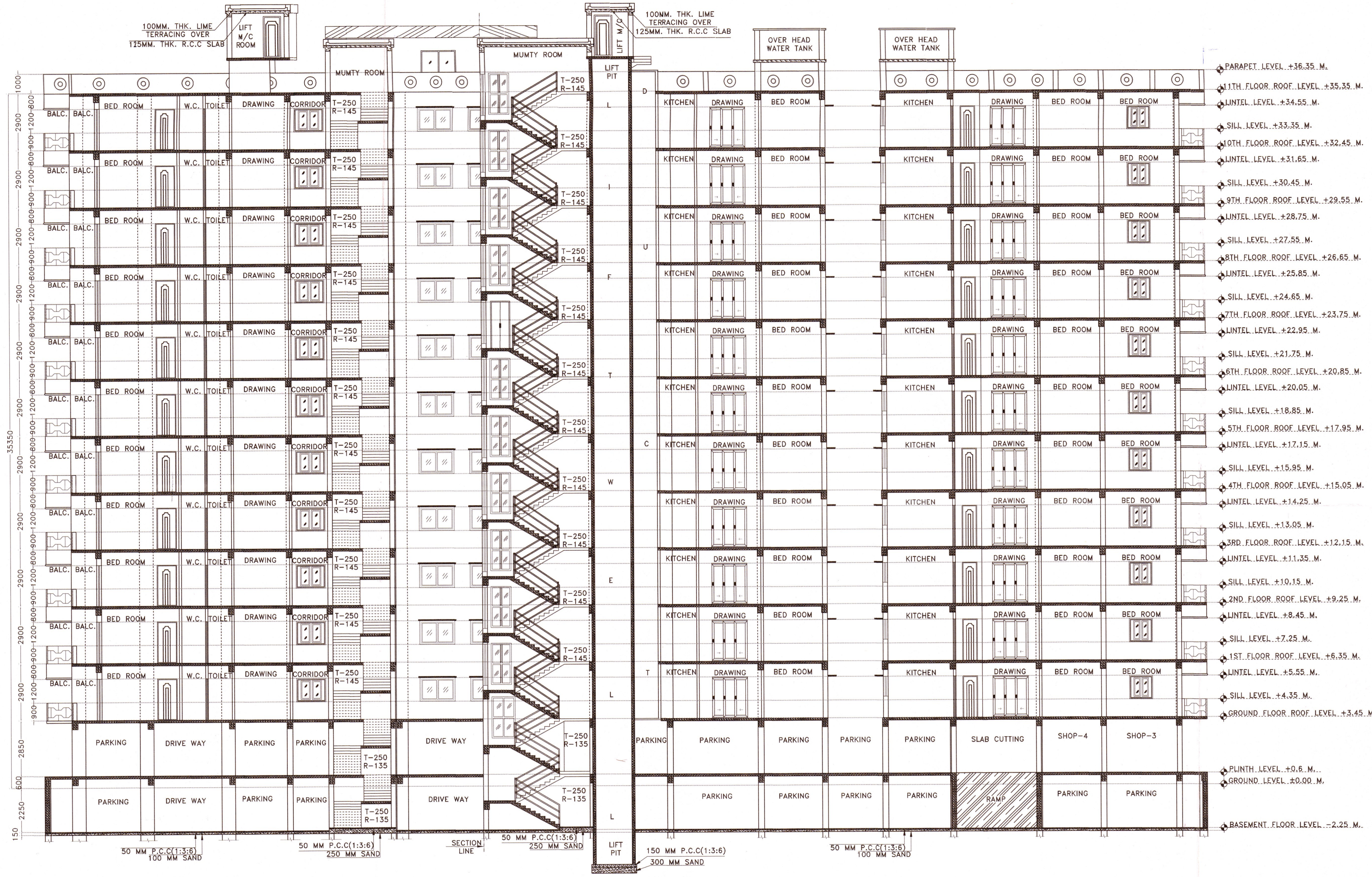
SECTION : X-X' SCALE: 1:100
